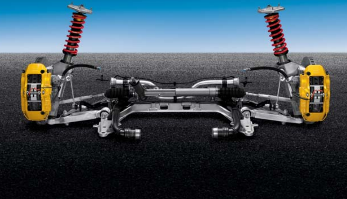
Essieu avant 911 GT3 doté de freins PCCB (Porsche Ceramic Composite Brake)
