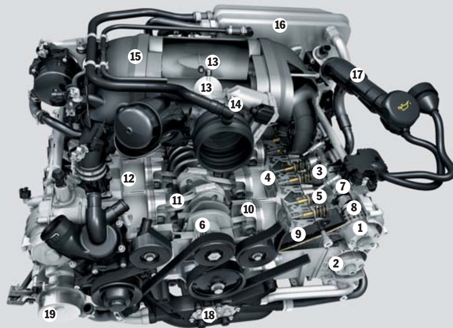
Moteur Boxer de 3,8 l de cylindrée de la 911 GT3
