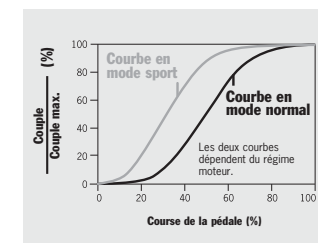
Courbe comparative de l'accélérateur électronique en mode normal et en mode sport
