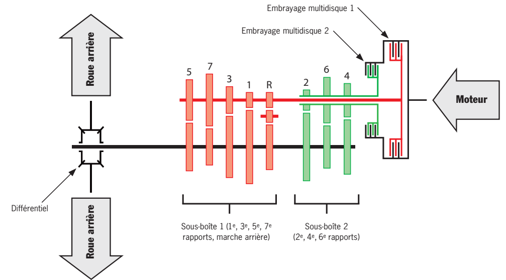
Principe de la boîte PDK
